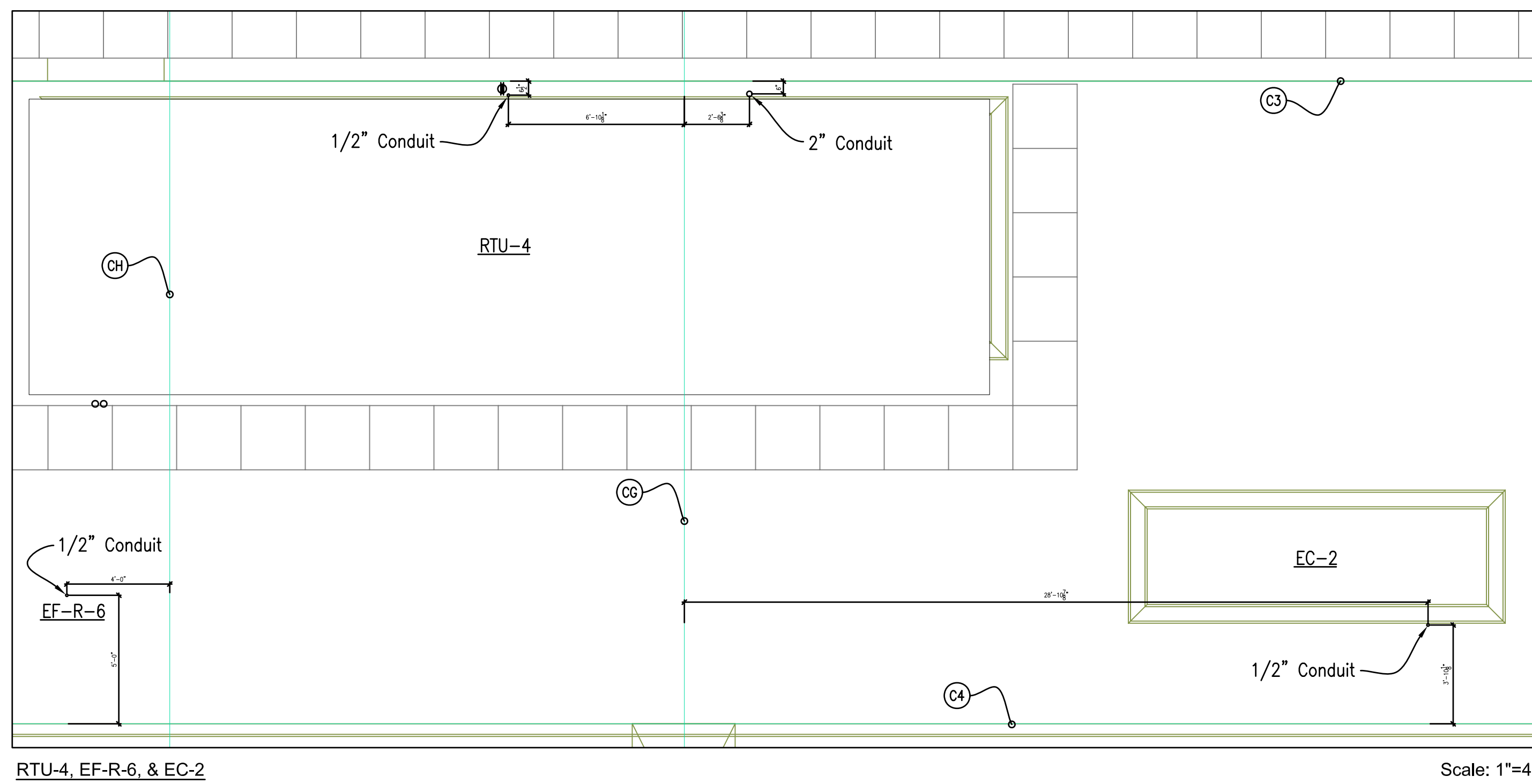
RTU-4, EF-R-6, & EC-2
