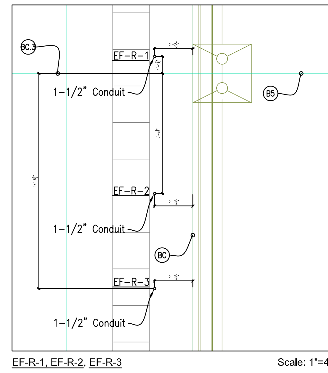
EF-R-1, EF-R-2, EF-R-3
